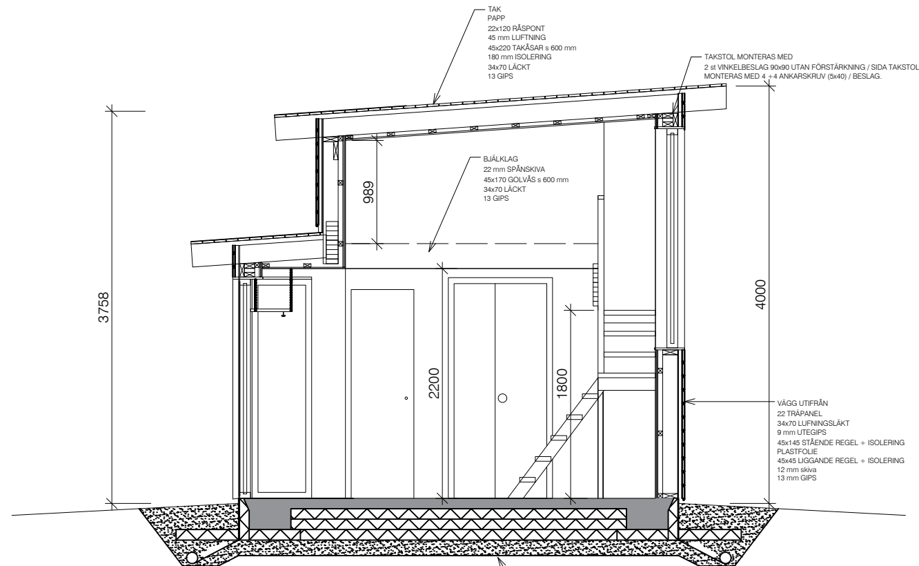
SEKTION A-A SKALA 1:50
