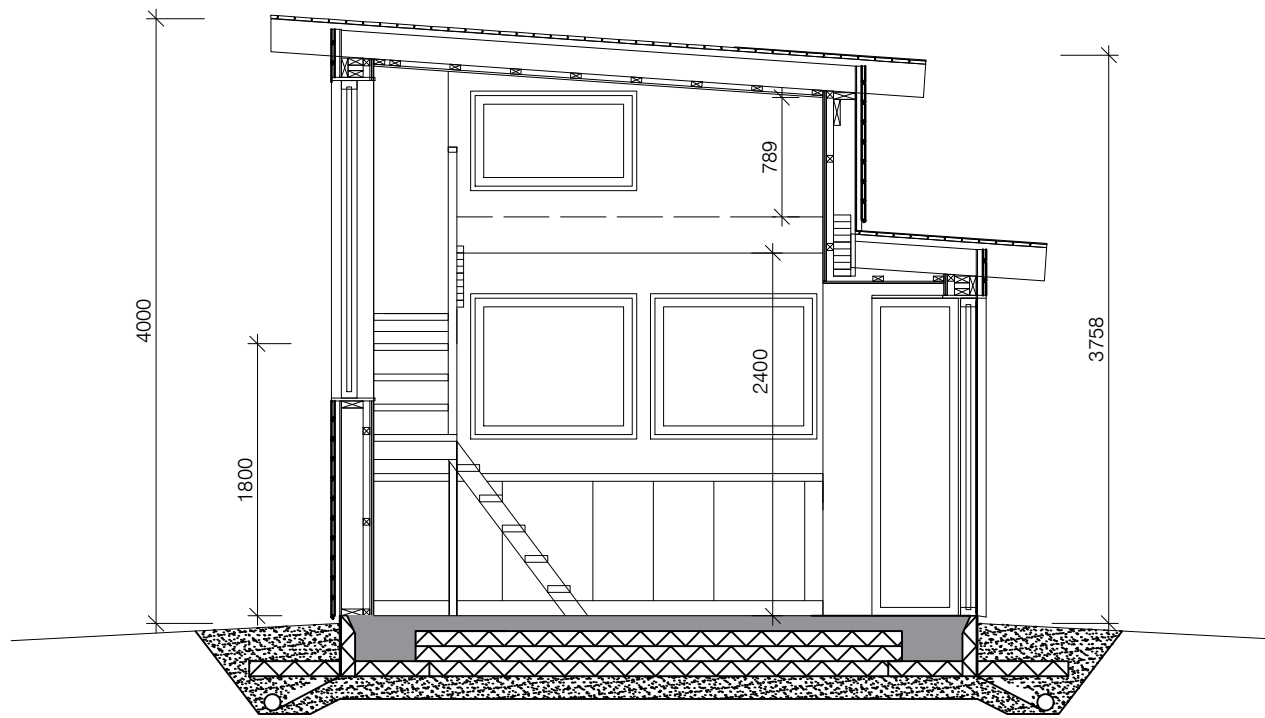
SEKTION B-B SKALA 1:50
