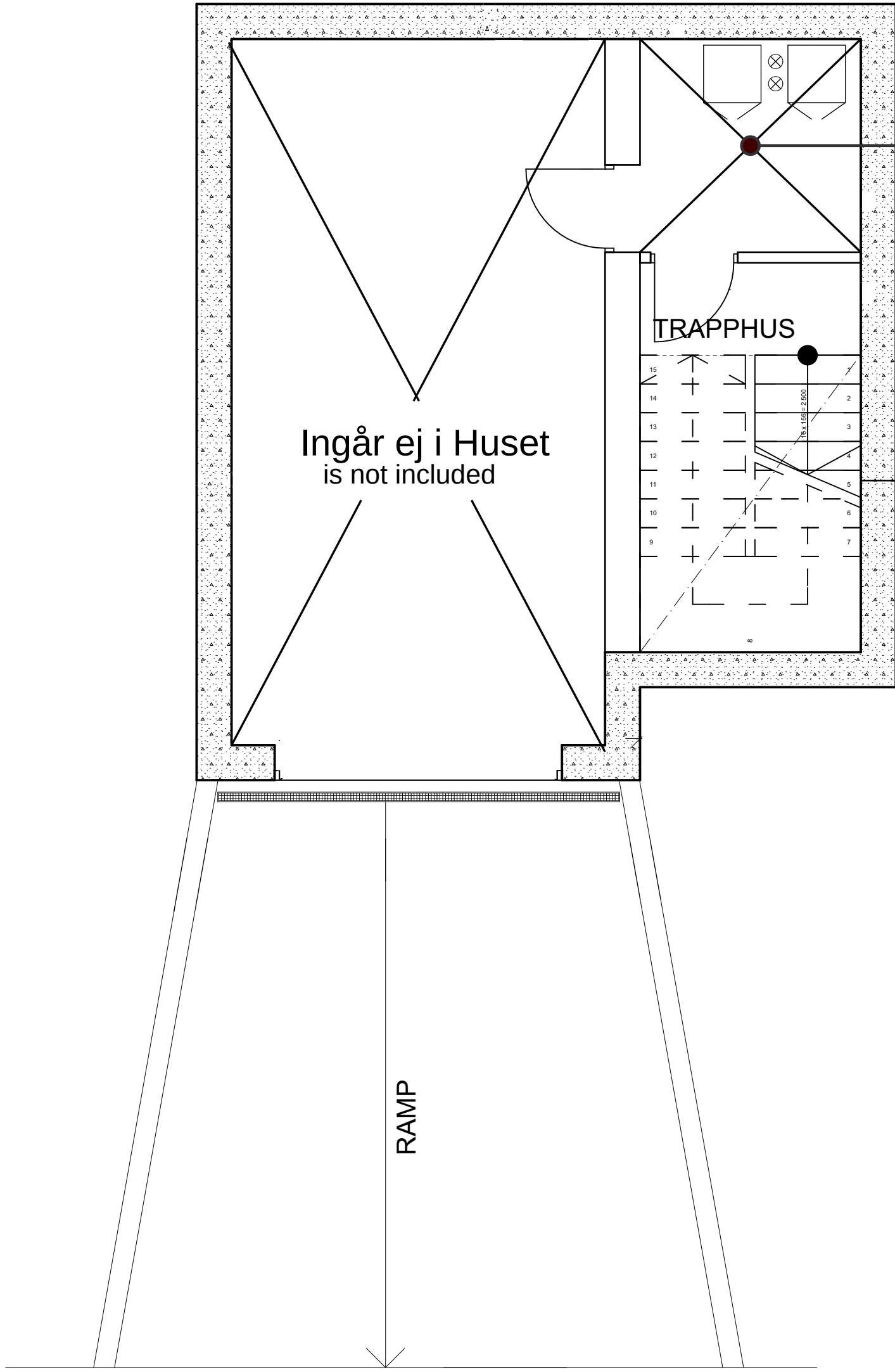
GARAGEPLAN
