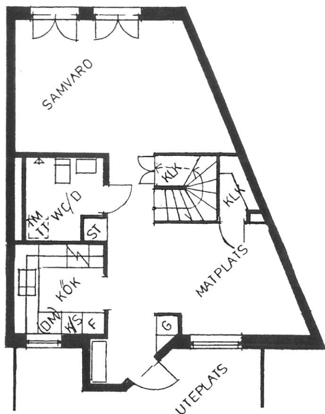
Bottenvåning
