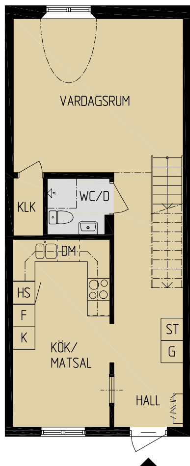
PLAN 1 (VÅNING 4)
