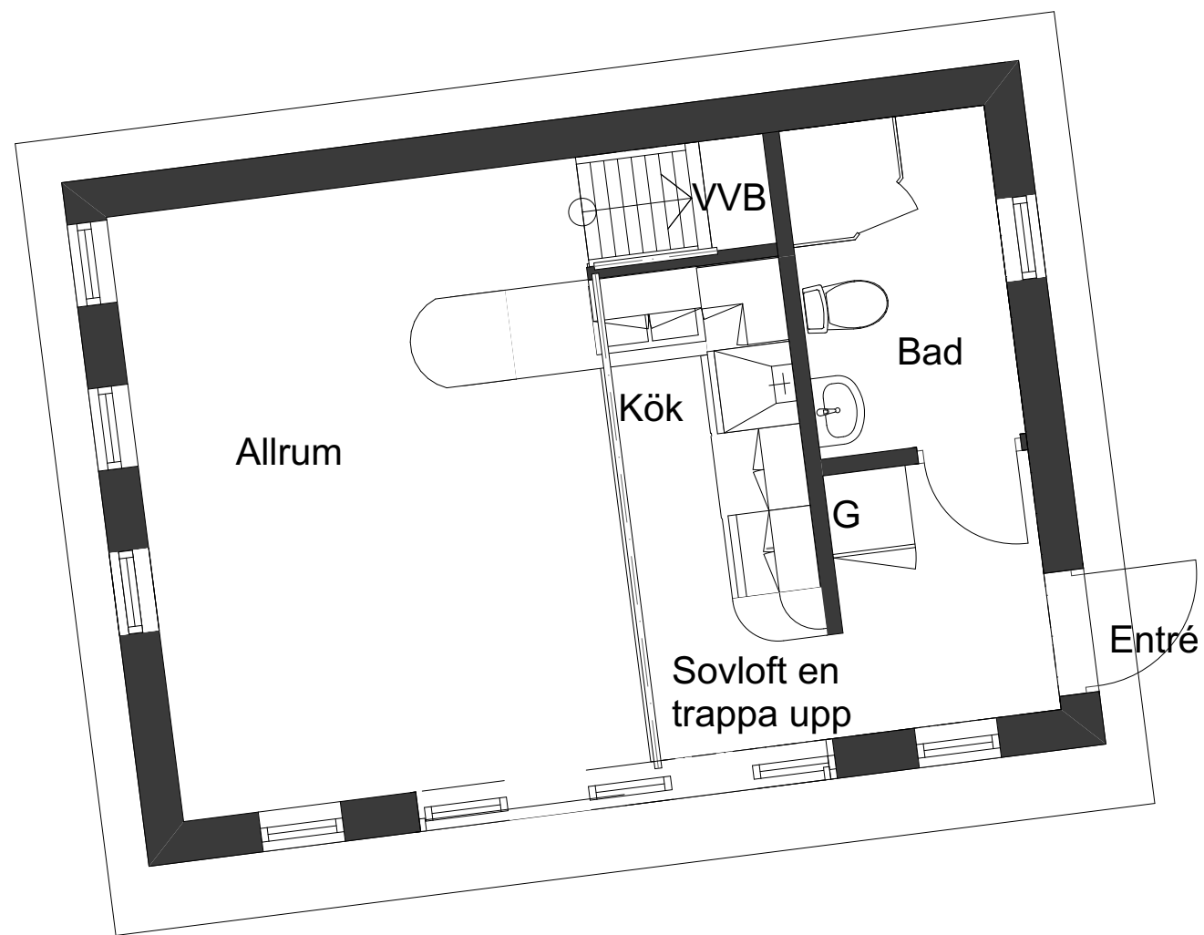
0. Entreplan med sovloft 1:50
