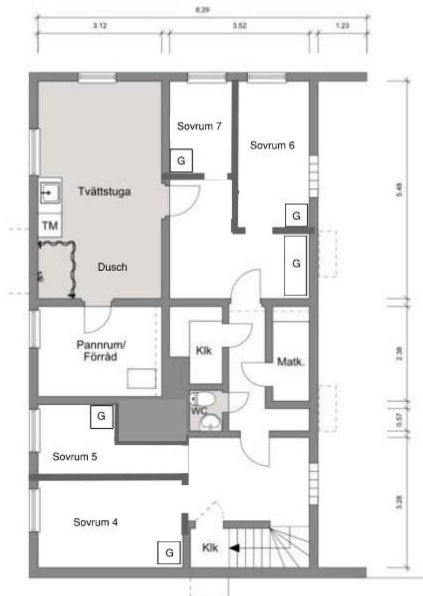
Källarplan
