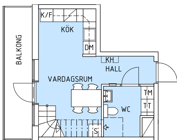
ENTRÉPLAN
