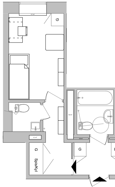
Plan 1 1:100
