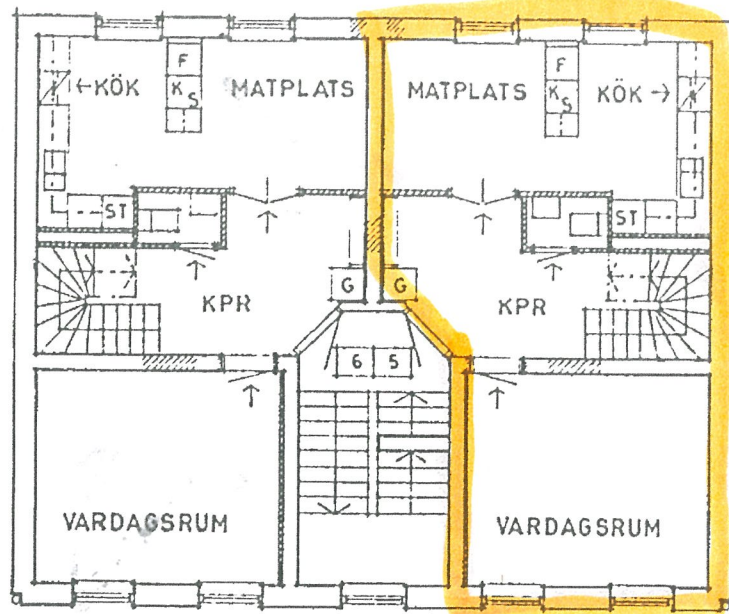
VÅNINGSPLAN 3
